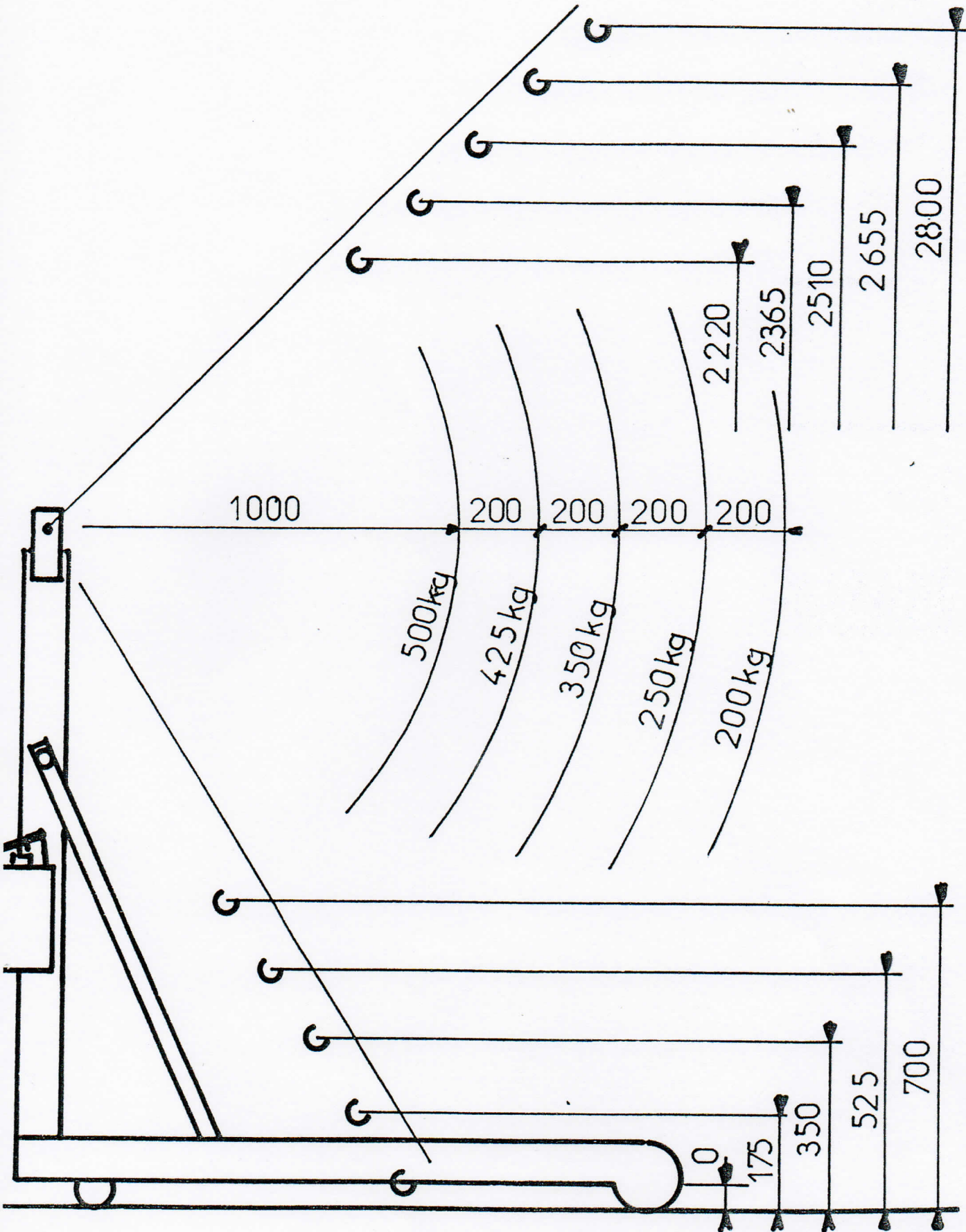
GRUE A 510 ( 500 kg ) ENCOMBREMENTS ET CHARGES
