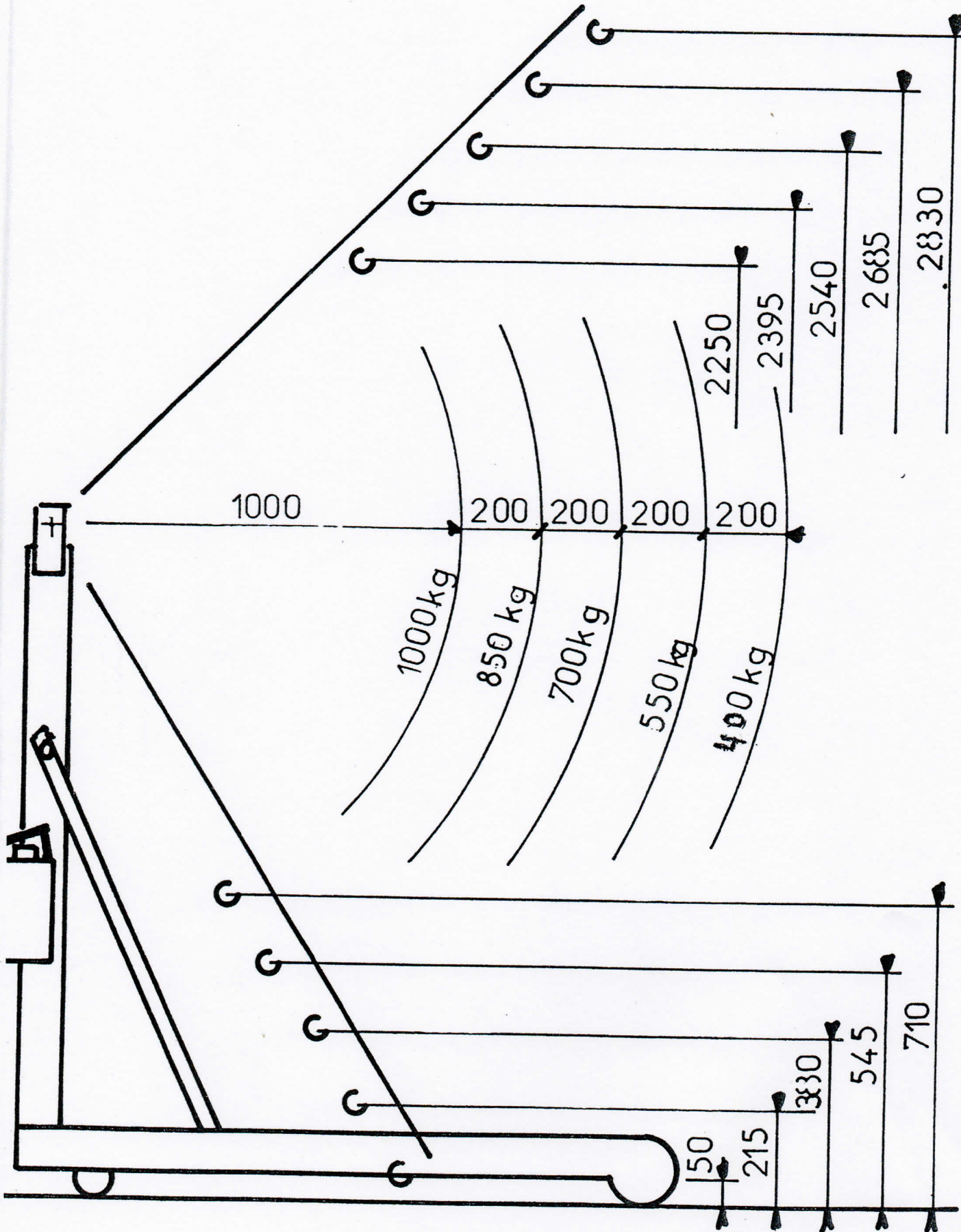
GRUE A 1010 ( 1000 KG ) ENCOMBREMENTS ET CHARGES
