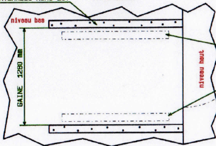
PAROIS LATERALES HORS LOT VUE DE DESSUS
