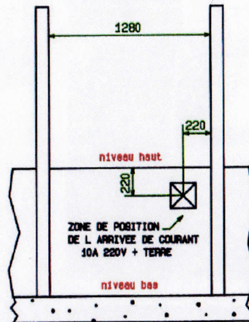
VUE DE FACE SUIVANT F
